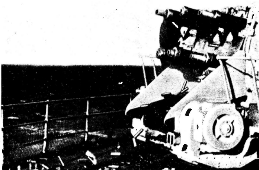
Montaje cuádruple de ametralladoras de 12 mm., instalado en los buques ingleses para hacer frente a los ataques rasantes de la aviación.
